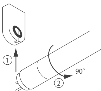
6、LEDランプの取付け
