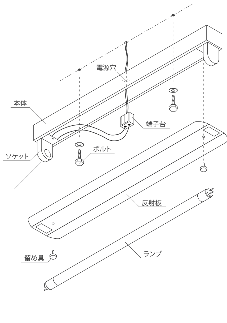
2、ソケットの取付け
